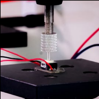
按键寿命测试 引进按键寿命试验机设备，测试产品按键的耐用程度和内部结构抗压强度。
